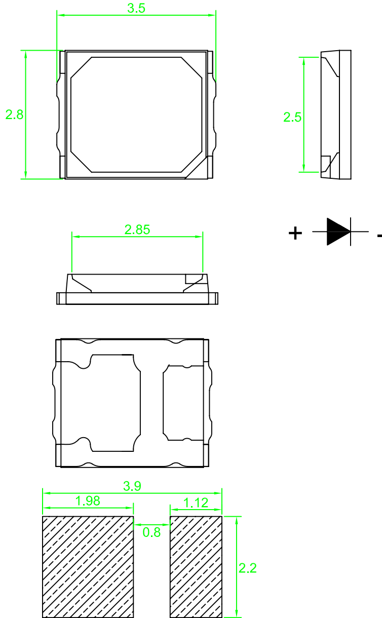
2835PCB图
